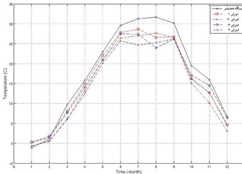
شکل ۱. دمای میانگین ماهانه شبیه‌سازی شده و ثبت همدید زنگان، ۱۹۹۰ میلادی. اجرای ۱: داده ورودی NNRP1، دقت مکانی 60 \times 60 کیلومتر - اجرای ۲: داده ورودی NNRP1، دقت مکانی 20 \times 20 کیلومتر - اجرای ۳: داده ورودی ERA40، دقت مکانی 60 \times 60 کیلومتر - اجرای ۴: داده ورودی ERA40، دقت مکانی 20 \times 20 کیلومتر
